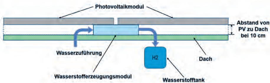
Projektskizze Wasserstoffherstellungsmodul
